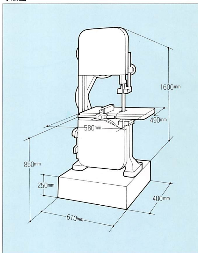
寸法図
